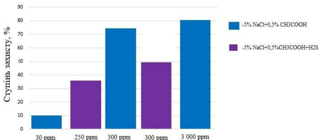
Рис. 1 Ступінь захисту сталі від корозії у розчині NACE без та з сірководнем з добавками екстракту берези.
