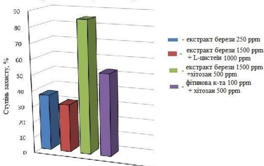
Рис. 2 Ступінь захисту сталі в сірководнево-вмісному середовищі за присутності екстракту листя берези та сумішей на основі цистеїну, хітозану та фітинової кислоти.
