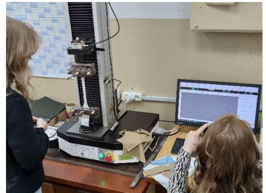
Рис. 3. Проведення лабораторних випробувань в умовах АДВЛ «Текстиль-ТЕСТ»
